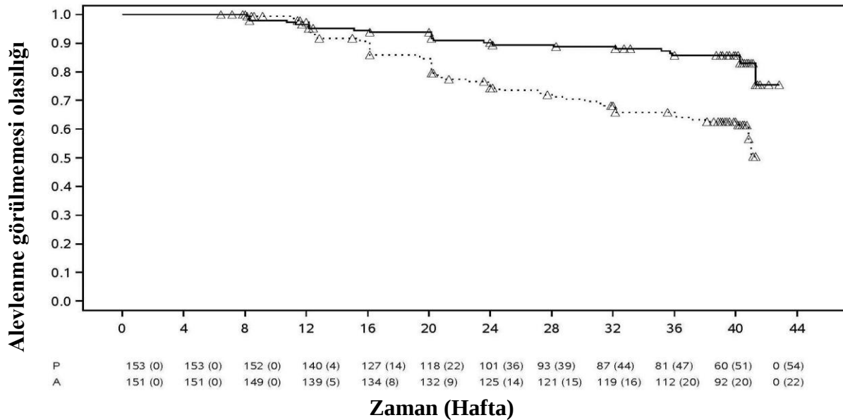
Şekil 1. nr-axSpA II Çalışmasında Alevlenme Zamanlamalarını Özetleyen Kaplan- Meier Eğrileri
