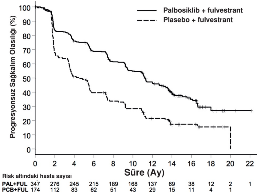
Şekil 2. Kaplan-Meier progresyonsuz sağkalım grafiği (araştırmacı değerlendirme, tedavi amaçlı popülasyon) – PALOMA-3 çalışması (Veri kesim tarihi 23 Ekim 2015)
